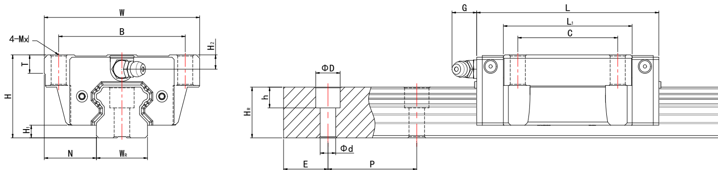
TIWINOK 品牌 11 系列高调心直线导轨 (俗称 HG) 法兰螺孔型滑块尺寸表
